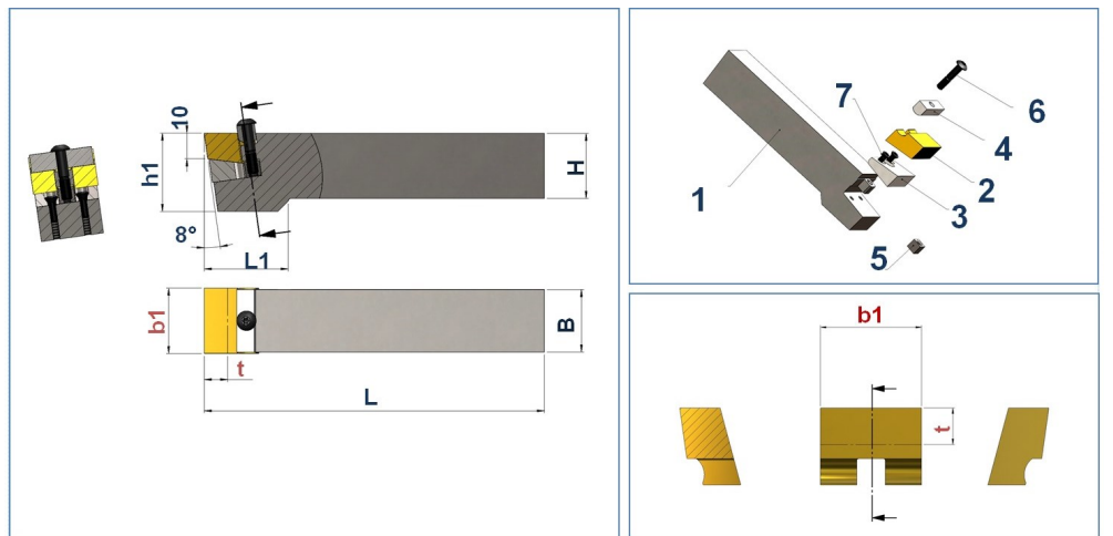
Werkzeughalter mit Innenkühlmittelzufuhr möglich Tool holders with internal coolant supply possible / Porte-outils avec des conduits d'arrosage internes possible
