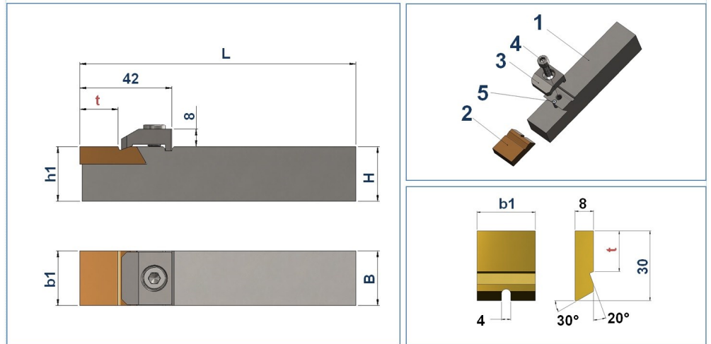
Werkzeughalter mit Innenkühlmittelzufuhr möglich Tool holders with internal coolant supply possible / Porte-outils avec des conduits d'arrosage internes possible
